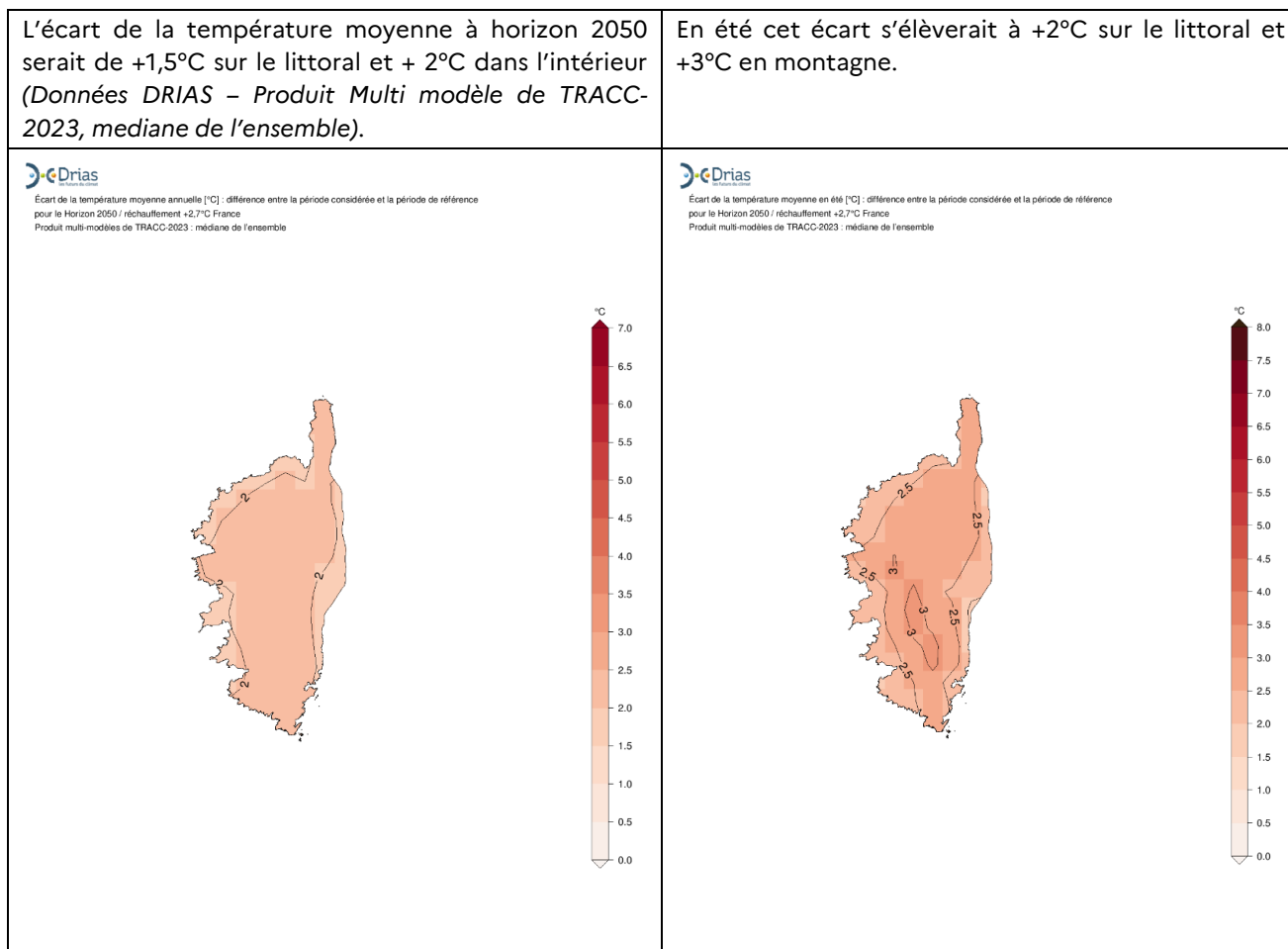
Illustration 25 : Ecart de la température moyenne annuelle et en été
