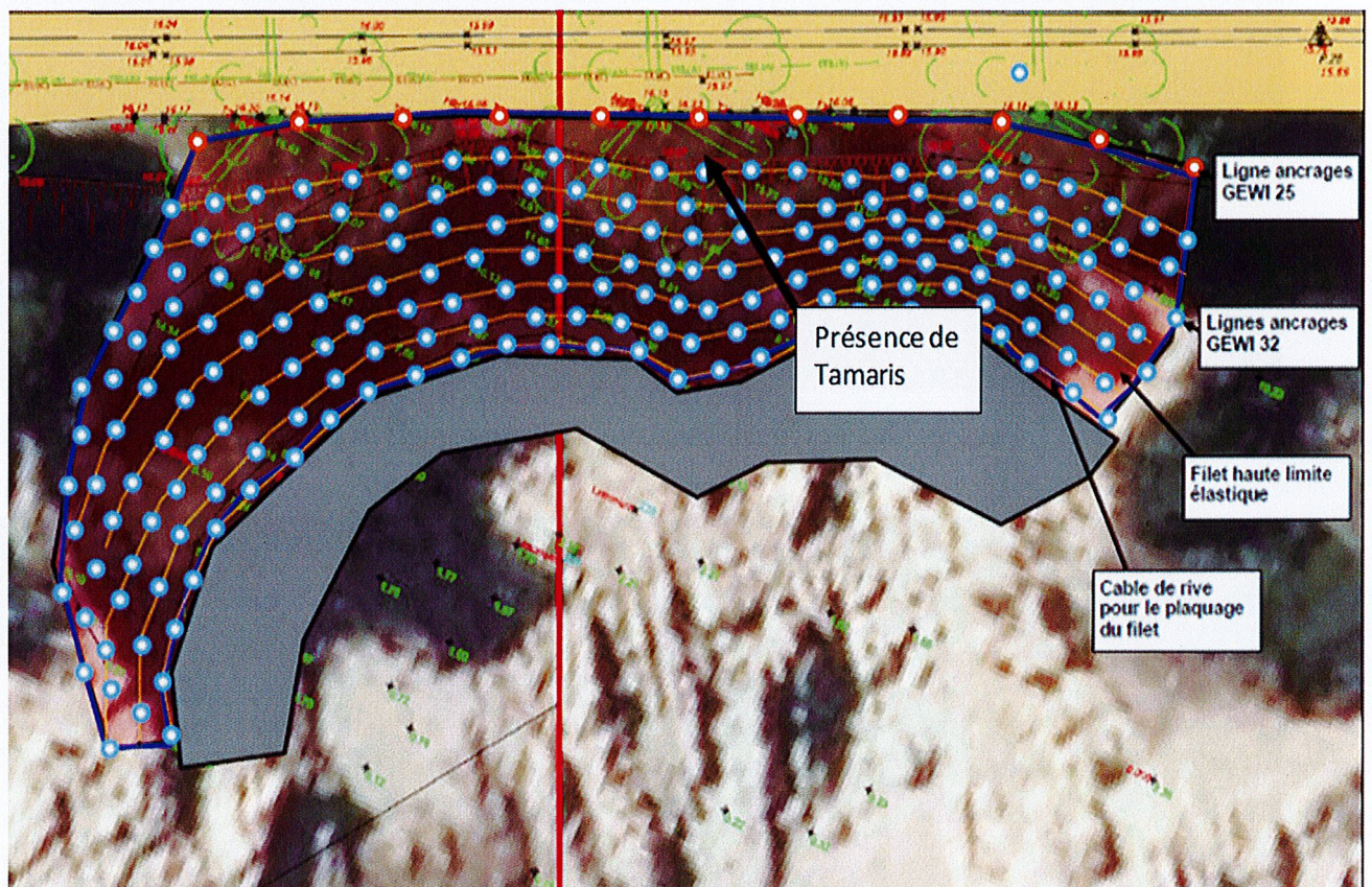
Vue en plan des travaux projetés
