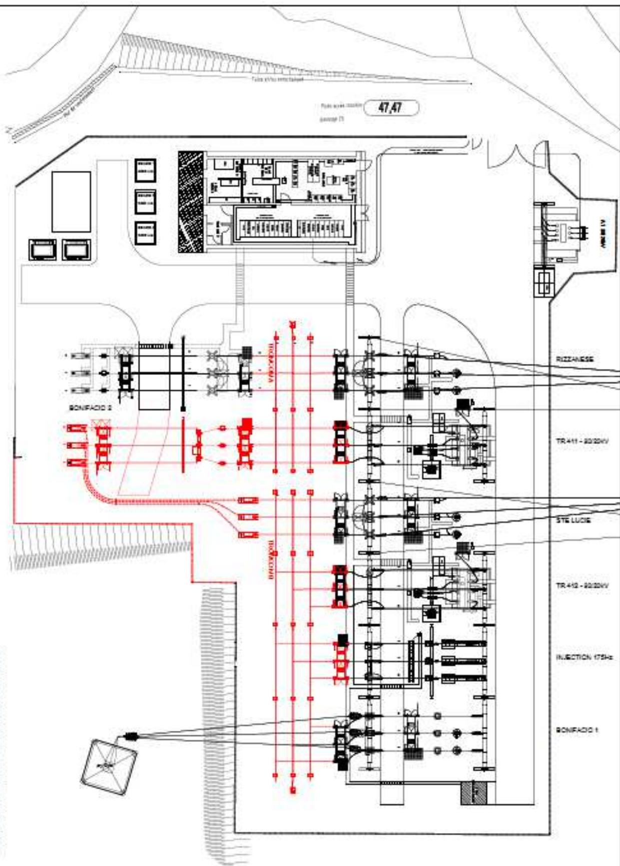
POSTE 90kV/20 kV DE PORTO VECCHIO SITUATION FINALE -version APD Minuée - VAE EN PLAN PROJET
