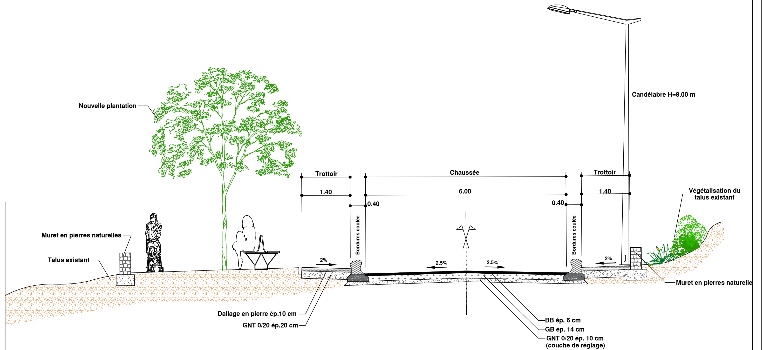
Profil A-A
