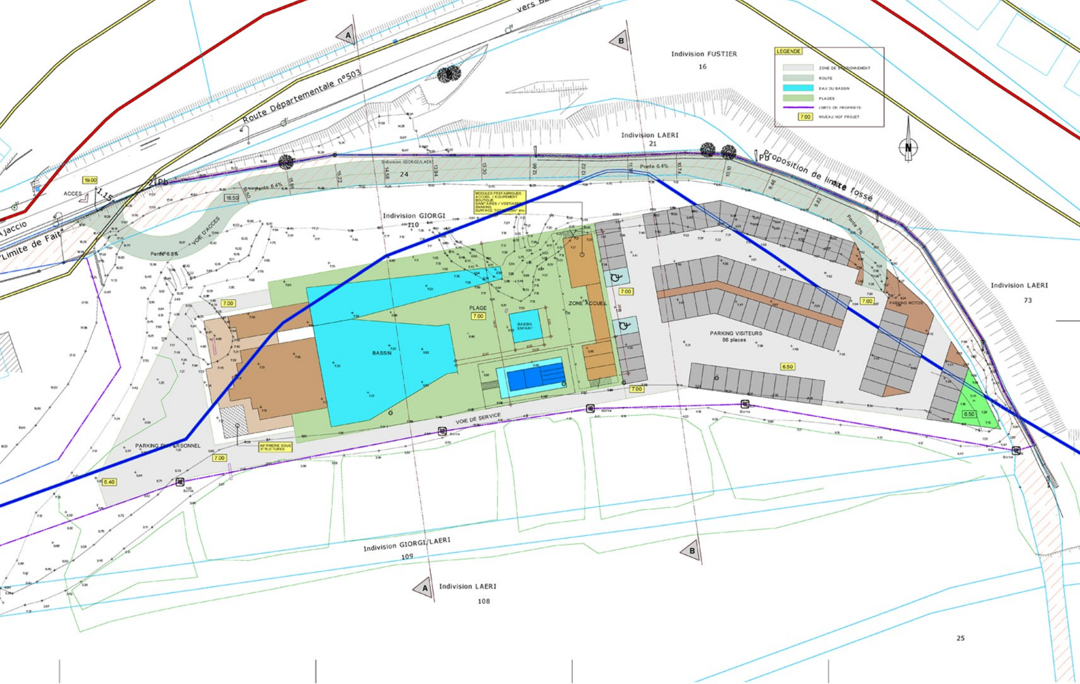
Annexe 4 : Projet Waterjump, évaluation au cas par cas des incidences du défrichement et du parking Plan d'implantation du projet
