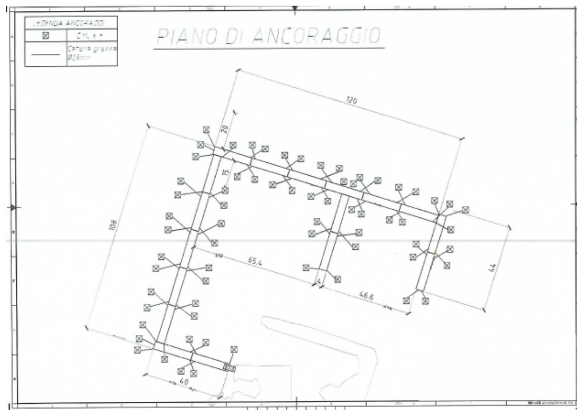
Plan d'ancrage
