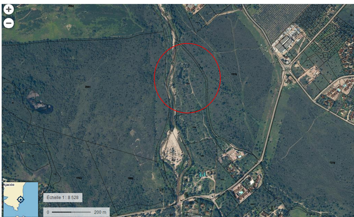
10. Site d'implantation de la Station d'épuration Coté Nord-Ouest
